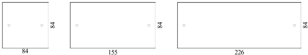
Серии Axiome, Tetra. Размеры пластин
