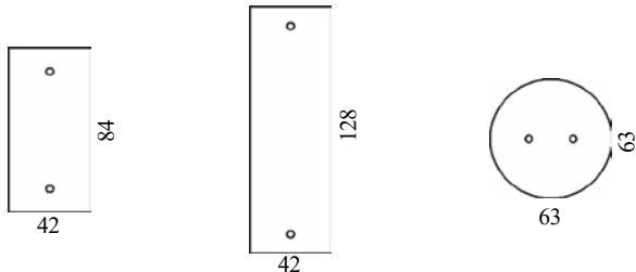
Серия Petite. Размеры пластин.
