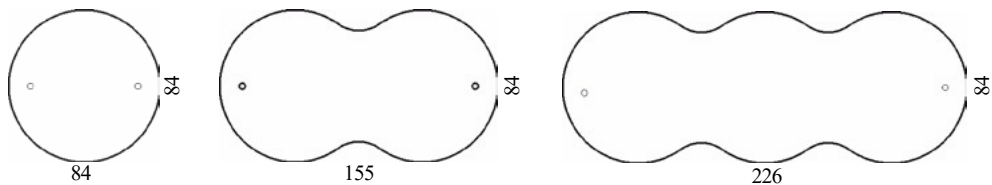
Серия Sphere. Размеры пластин
